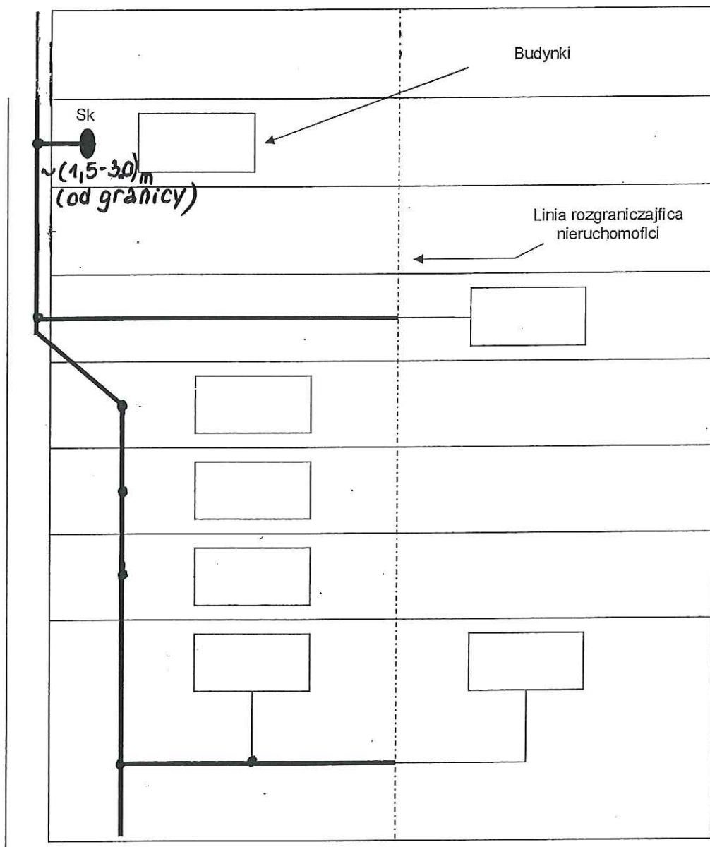
Rysunek 1. Kanalizacja grawitacyjna Pogrubione odcinki sieci stanowi element kwalifikowalny.
